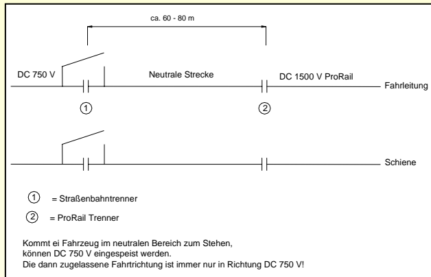
Systemwechselstelle 750V DC auf 1500V DC
