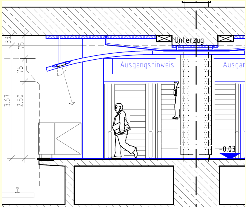
Schnittdarstellung mit neuer Deckenkonstruktion in der Fahrebene Quelle: APB-Architekten
