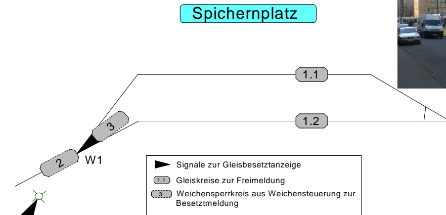
Prinzipbild der Gleisbesetztanzeige
