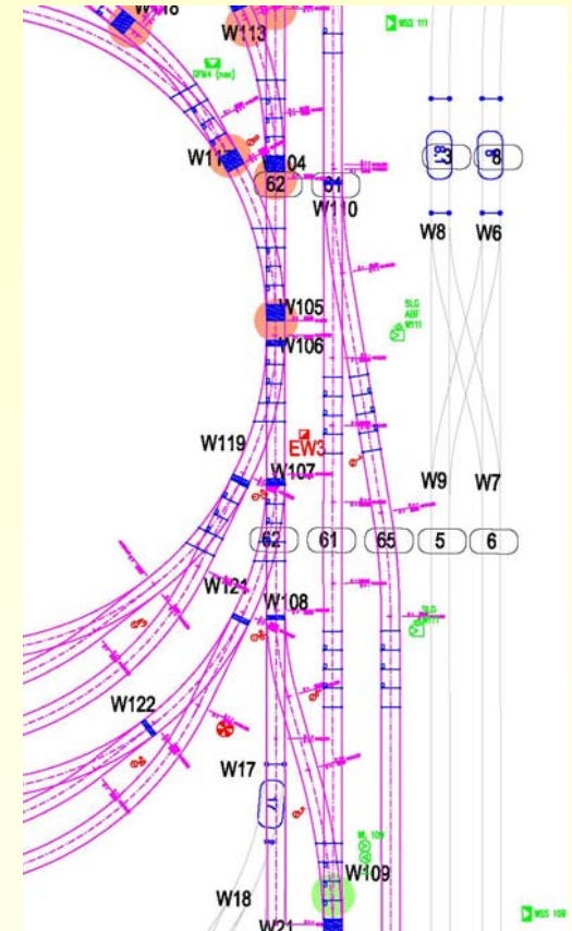
Auszug zum Gleisschemaplan
